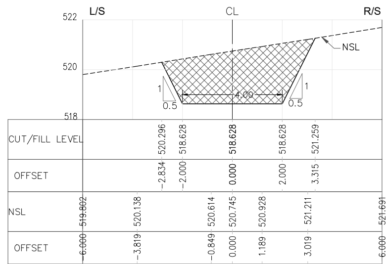
RD=2+800.000
