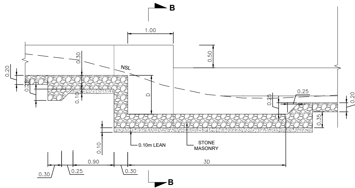
CANAL FALL LONGITUDINAL SECTION A-A
