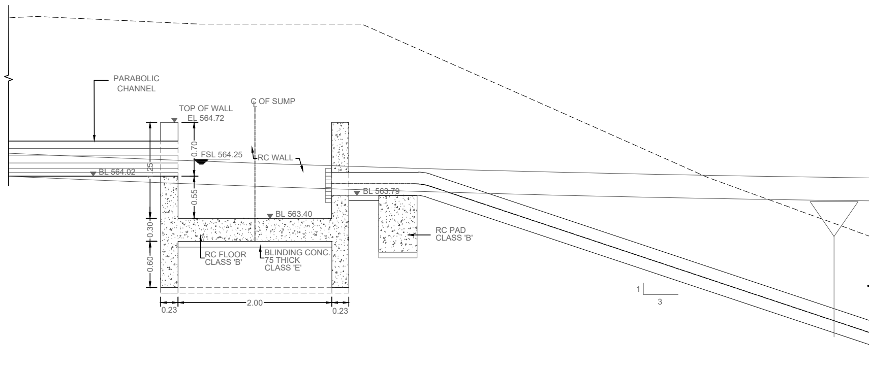
SECTION A-A
