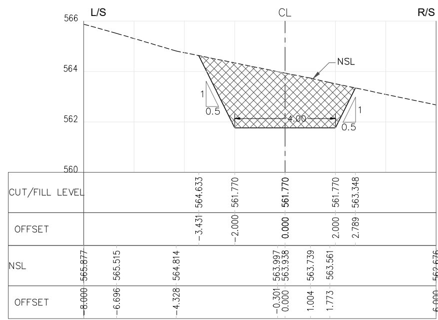
RD=1+550.000
