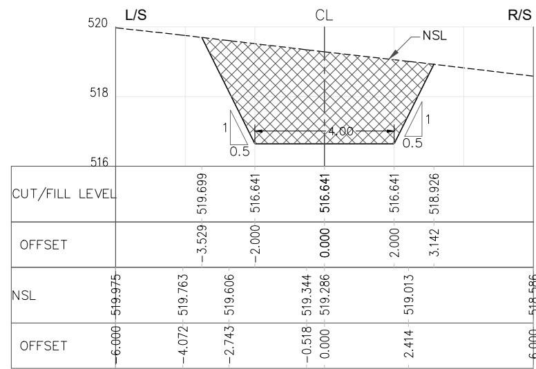
RD=3+050.000
