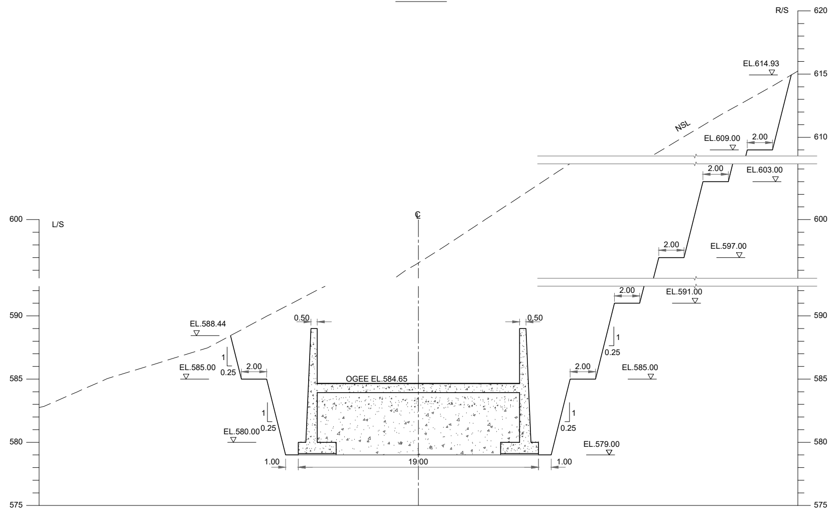
RD 0+000
