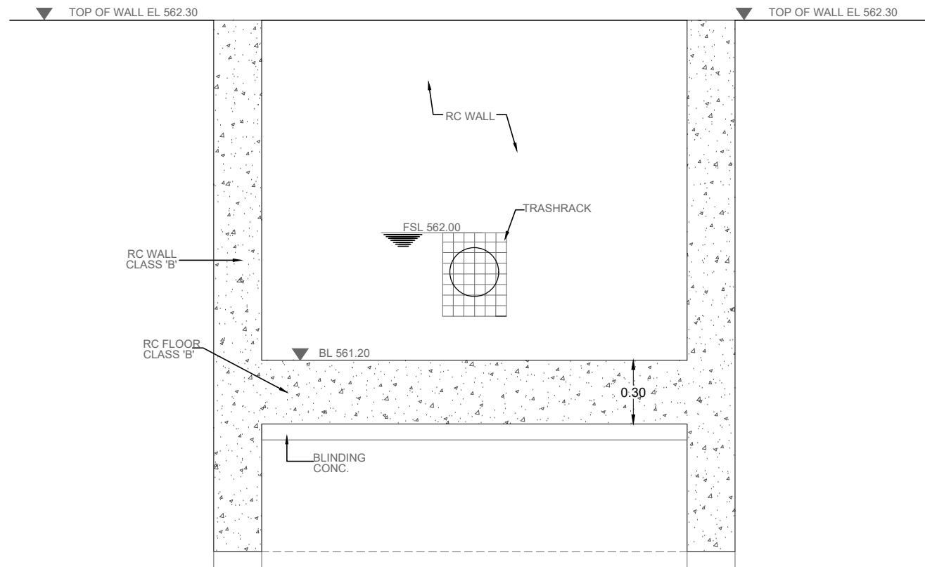
SECTION D-D
