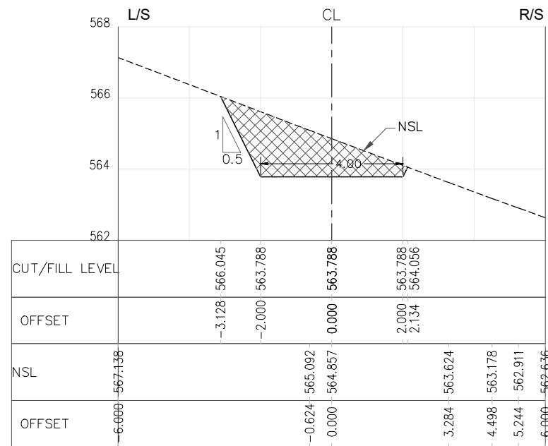
RD=1+350.000
