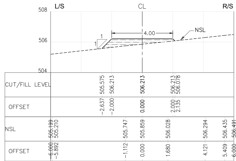
RD=3+400.000
