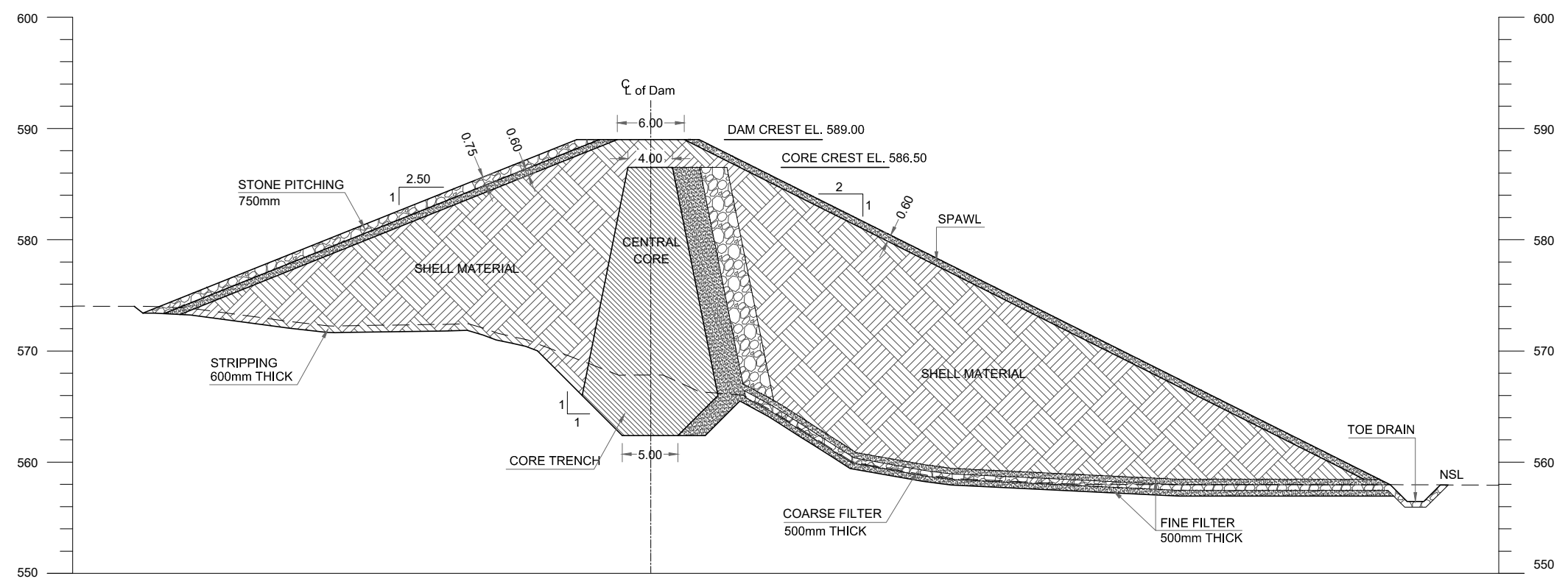
RD 0+040
