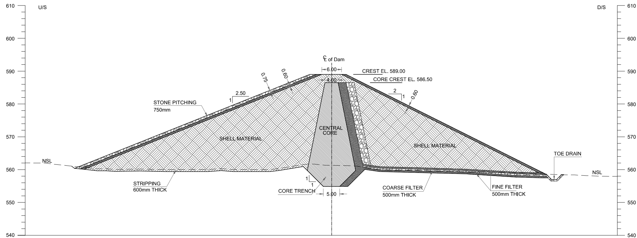
RD 0+140
