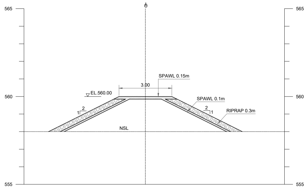
A-A
