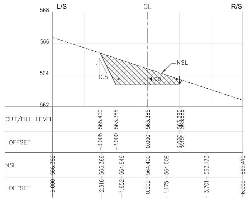
RD=1+300.000
