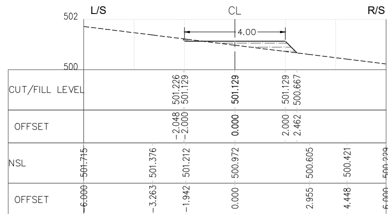
RD=3+550.000
