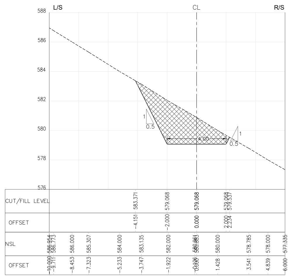
RD=0+200.000
