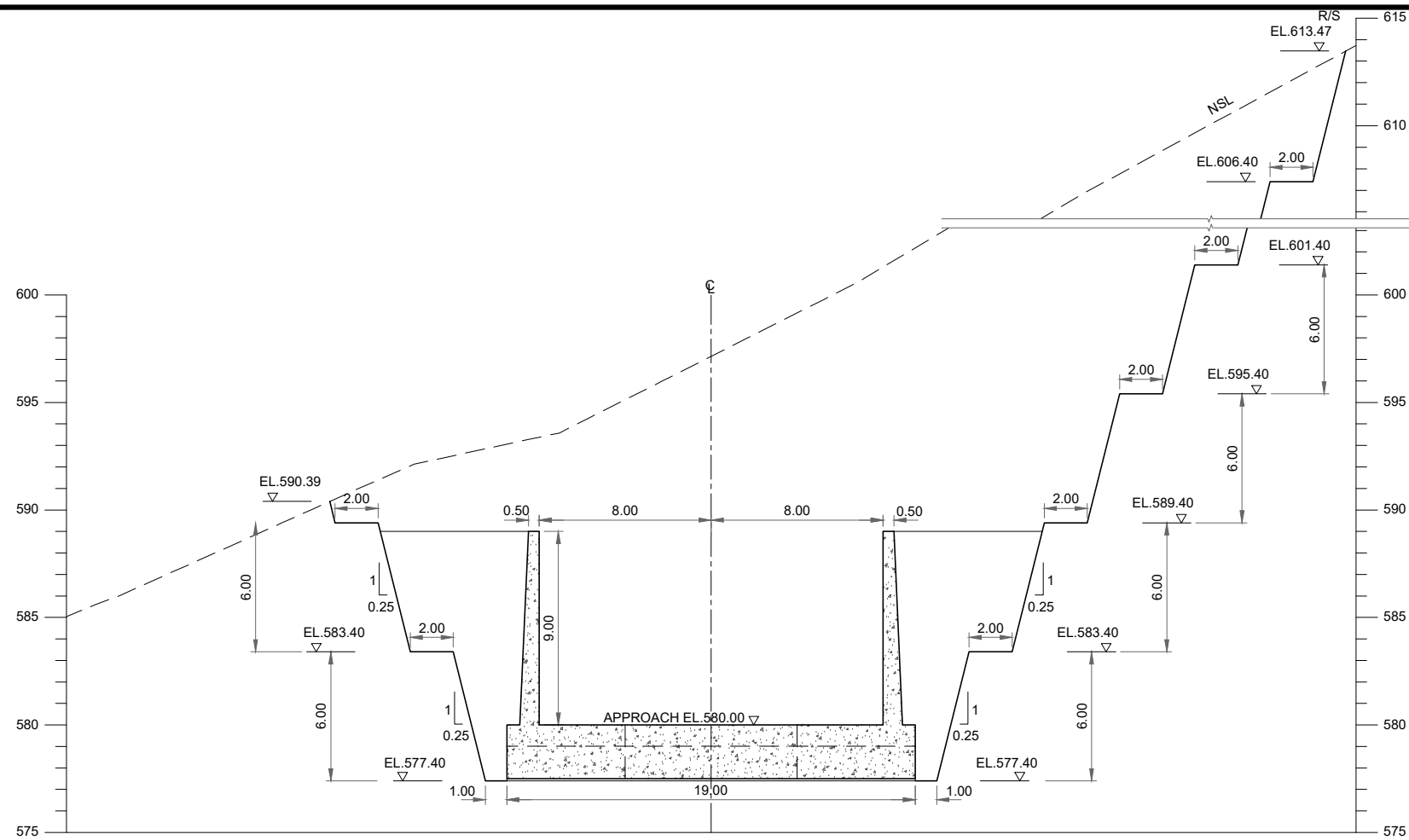
RD 0-010
