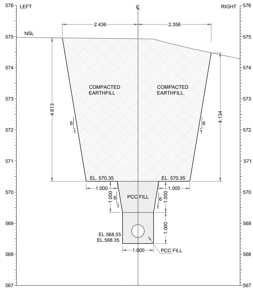
RD 0+030
