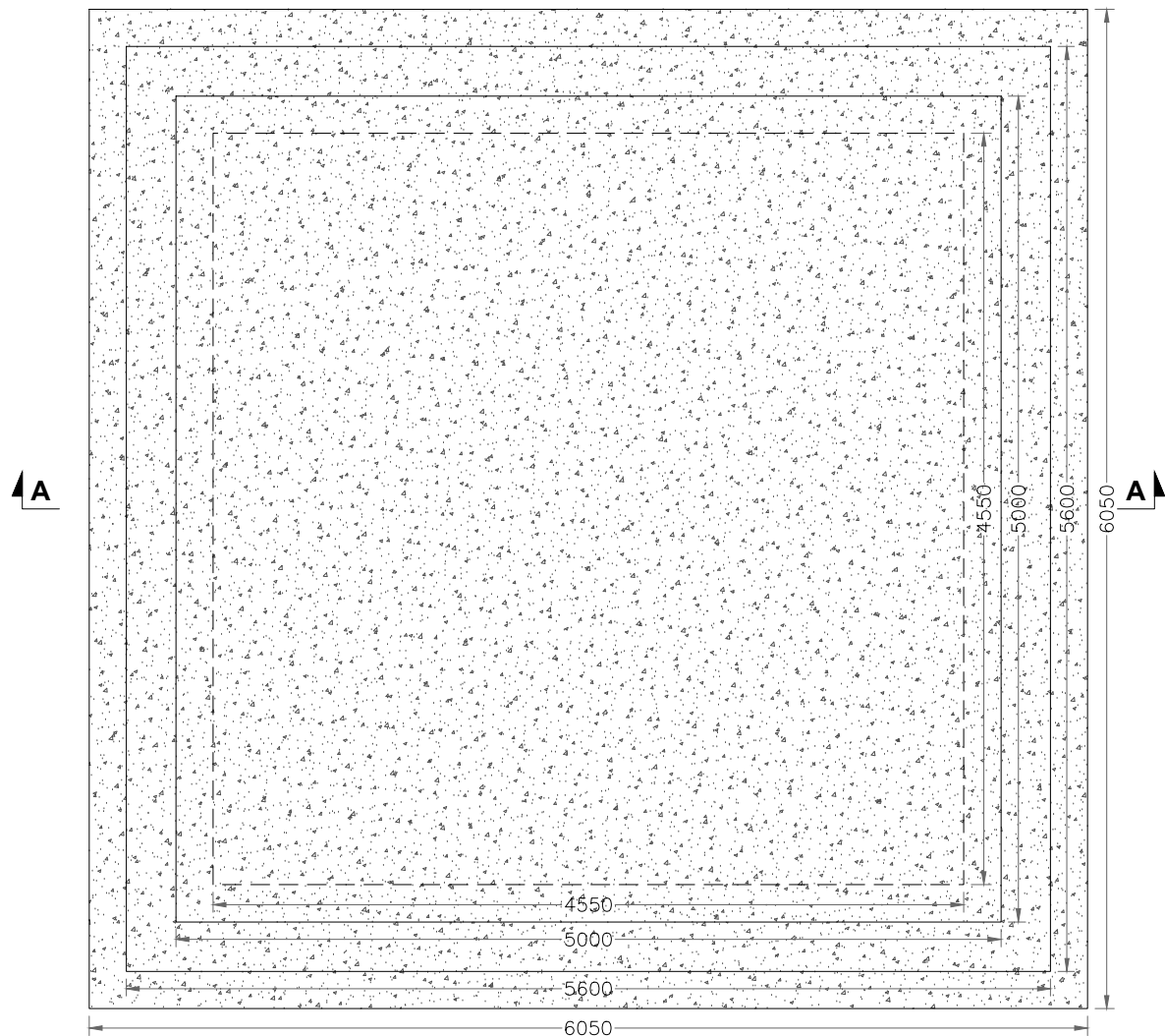
PLAN SCALE: 1:70
