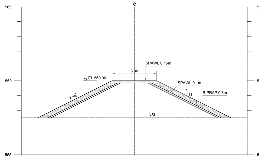
D-D
