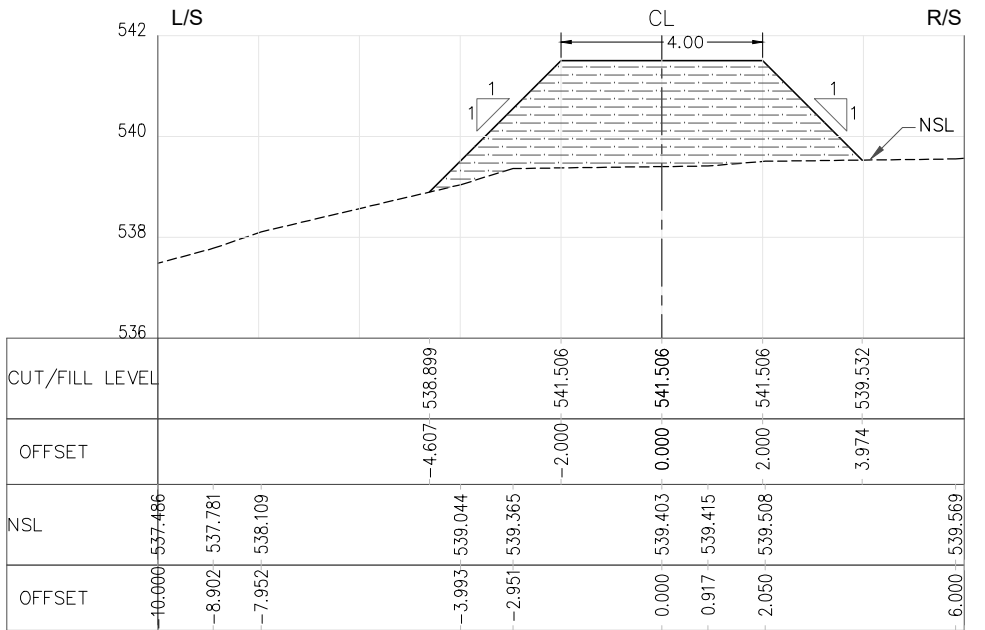
RD=2+100.000
