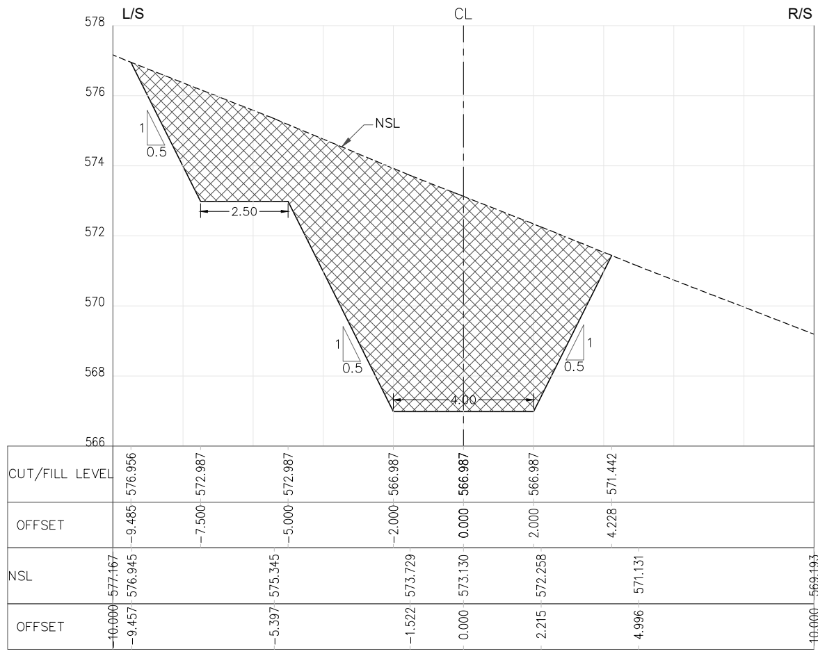
RD=0+900.000
