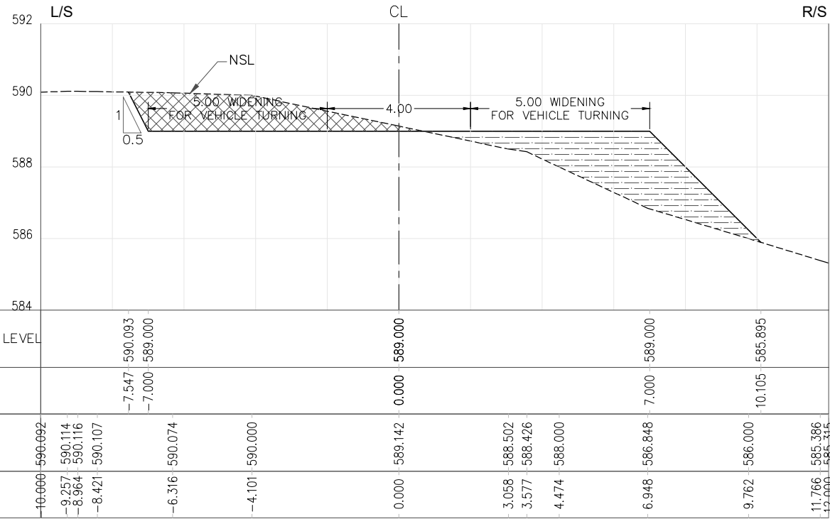
RD=0+000.000
