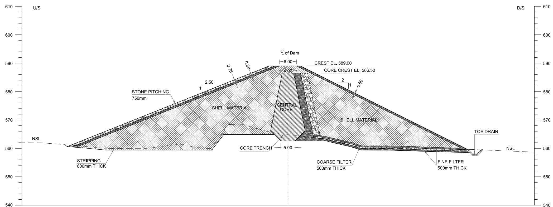
RD 0+160
