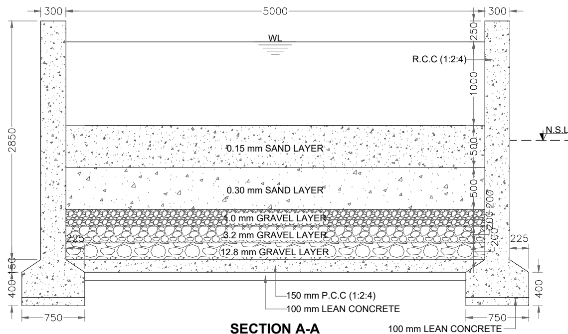
SECTION A-A SCALE: 1:70
