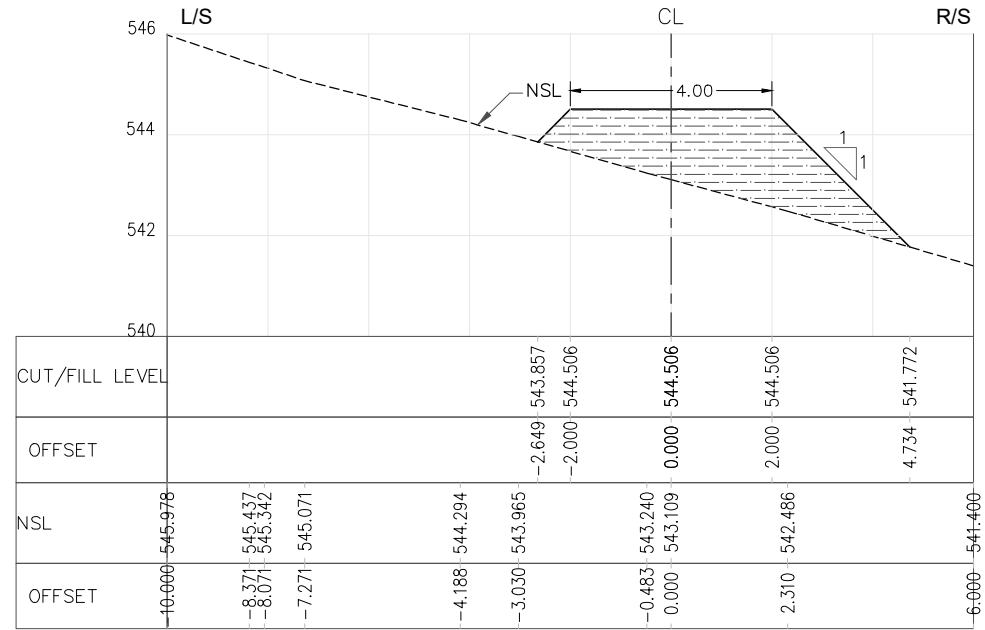
RD=2+050.000
