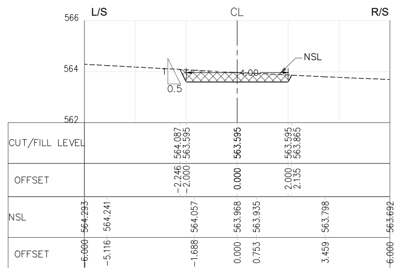
RD=1+400.000
