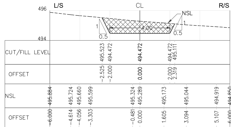
RD=3+750.000
