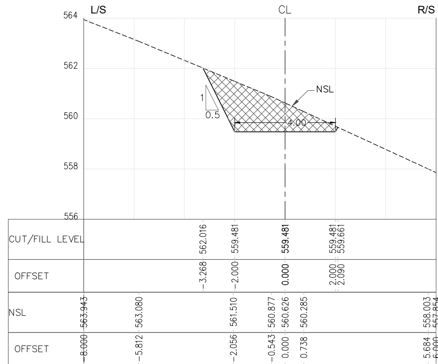
RD=1+650.000
