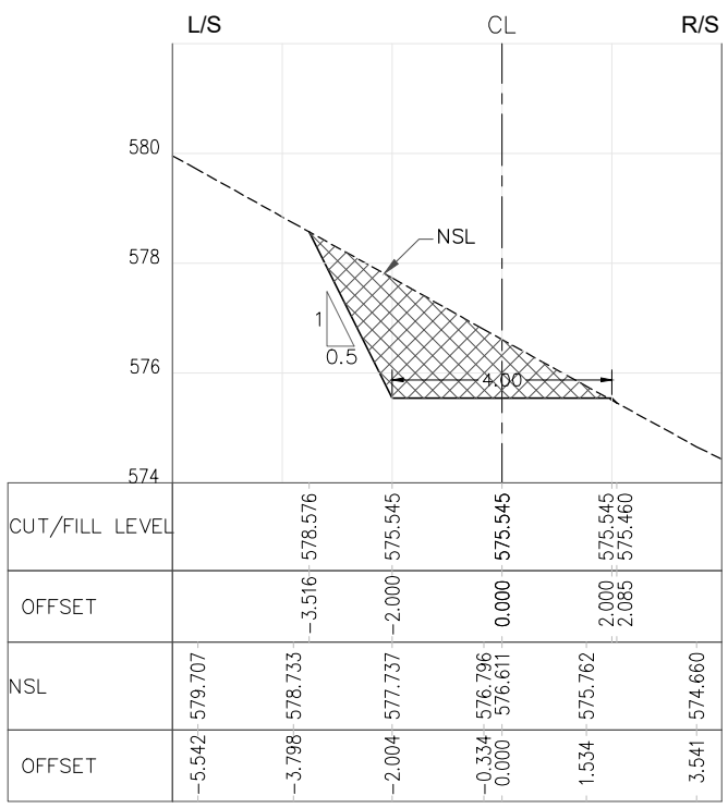
RD=0+600.000
