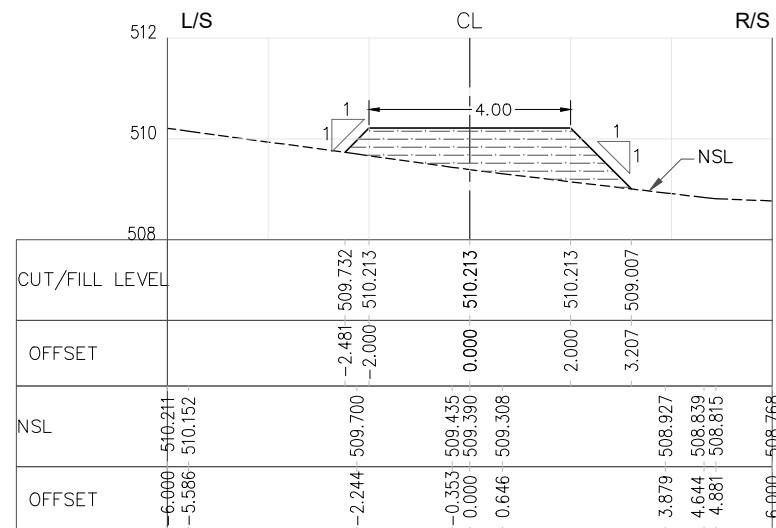
RD=3+250.000
