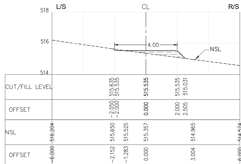
RD=2+950.000
