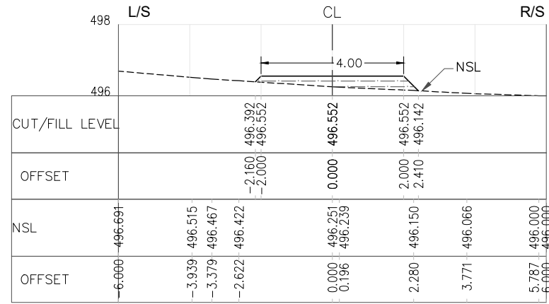
RD=3+650.000
