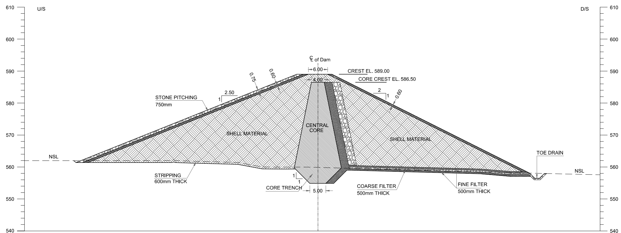
RD 0+080
