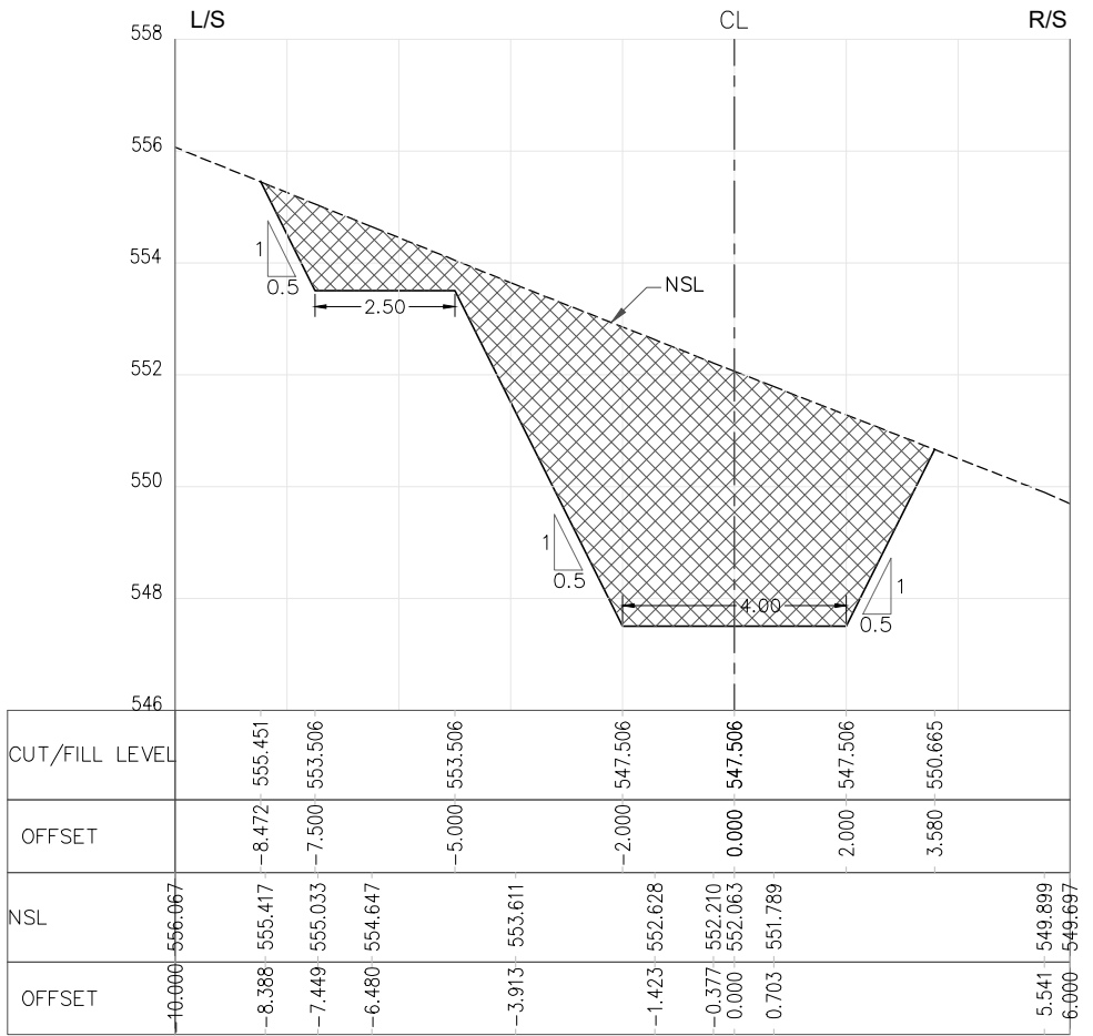
RD=2+000.000
