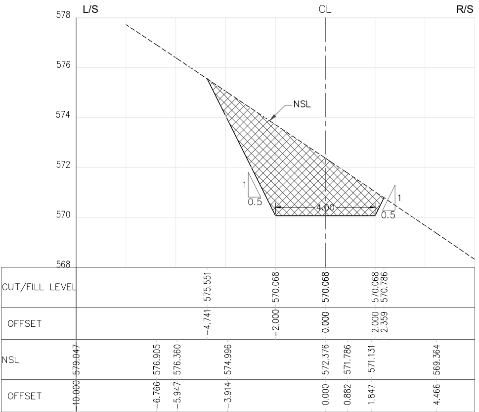
RD=0+700.000
