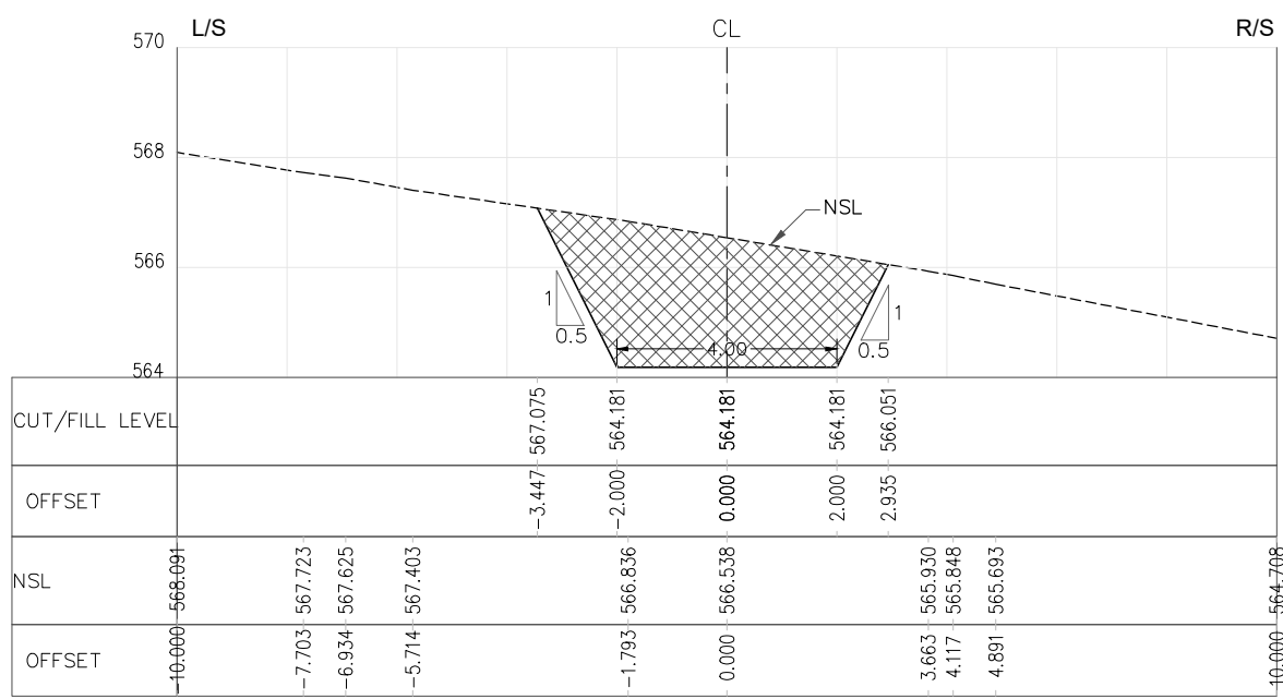
RD=0+800.000
