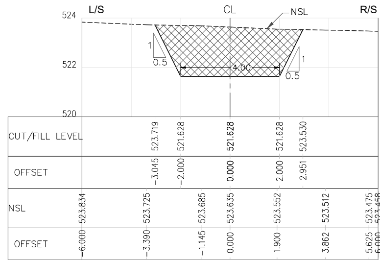
RD=2+750.000
