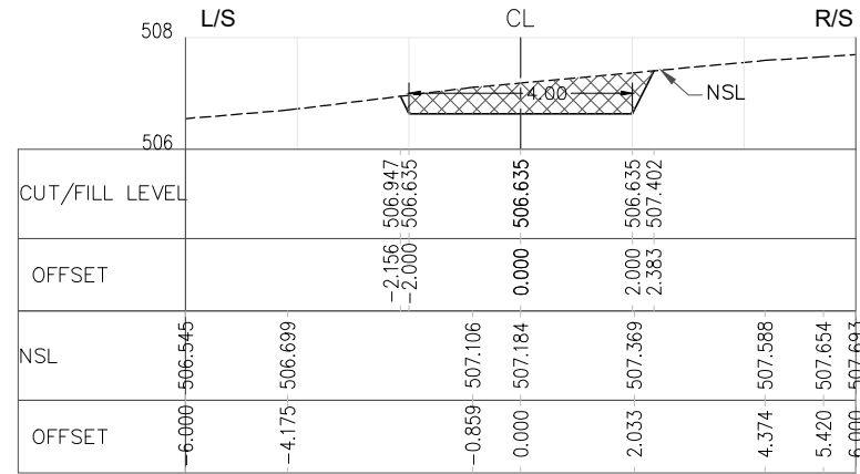
RD=3+350.000
