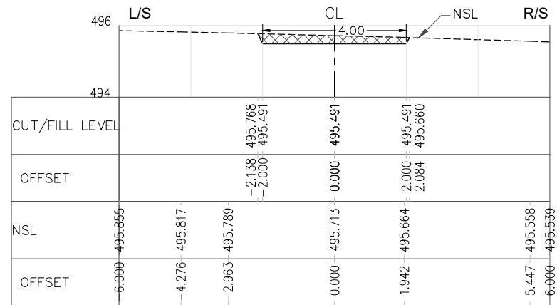
RD=3+700.000
