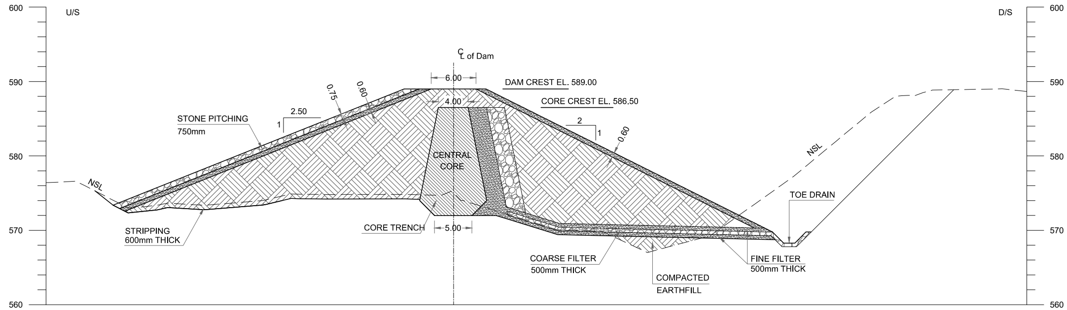
RD 0+240
