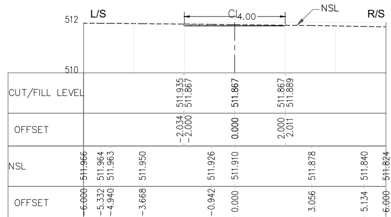
RD=3+200.000
