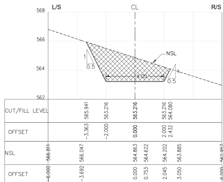
RD=1+450.000
