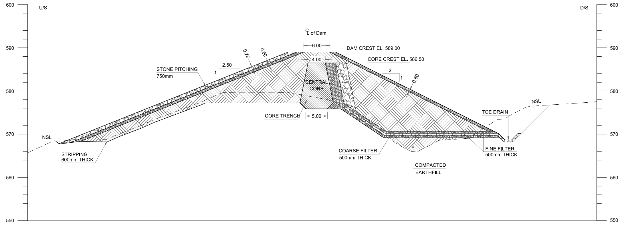
RD 0+220
