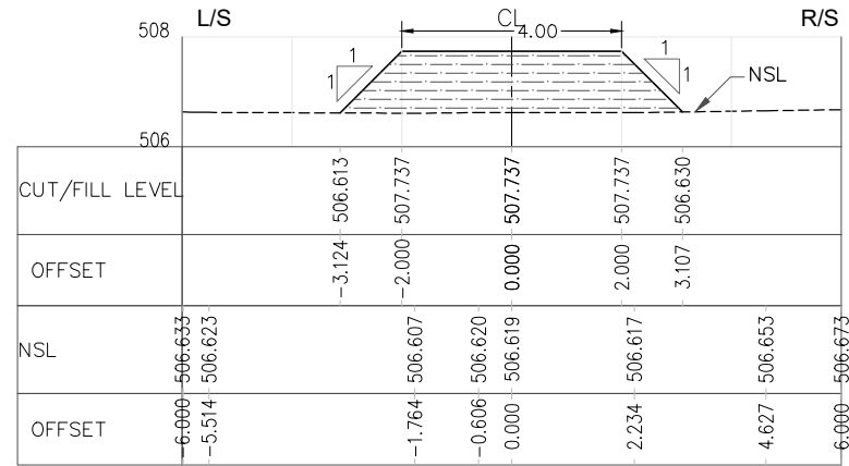
RD=3+300.000
