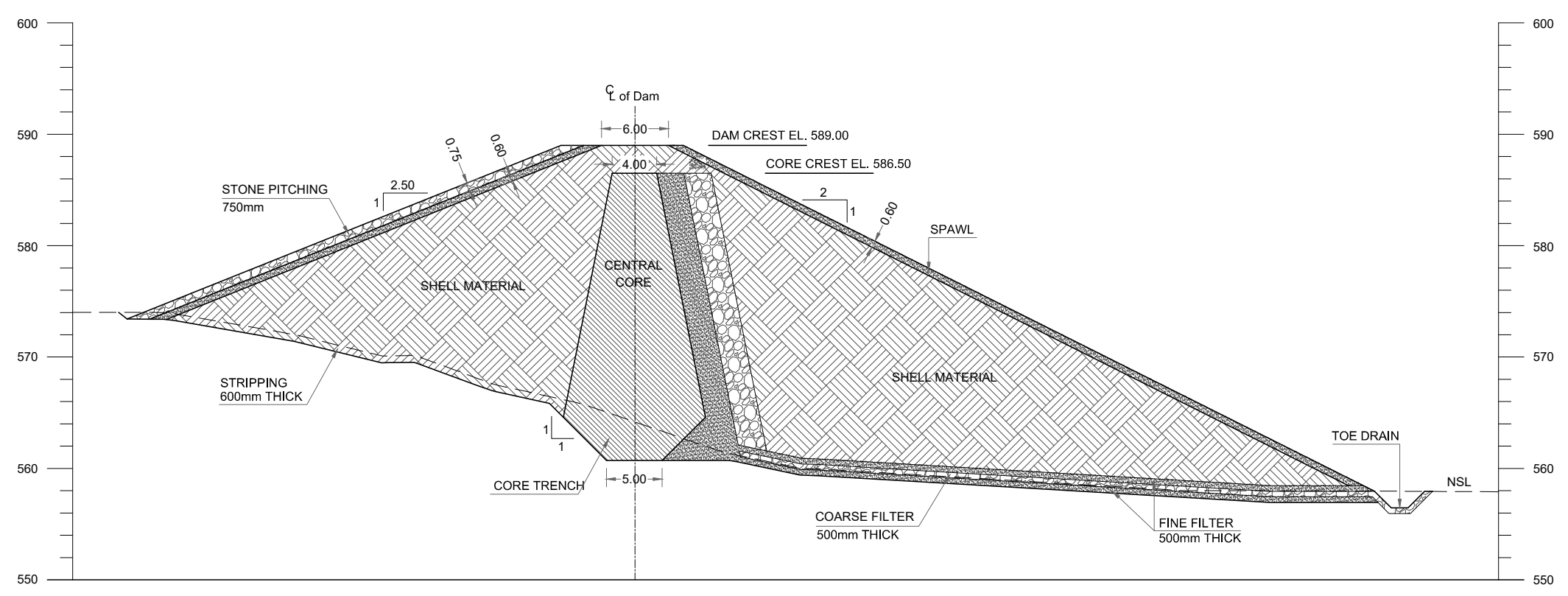
RD 0+050
