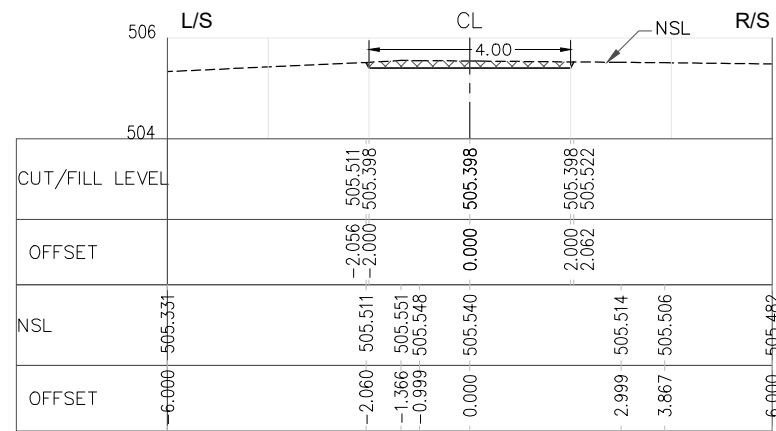
RD=3+450.000
