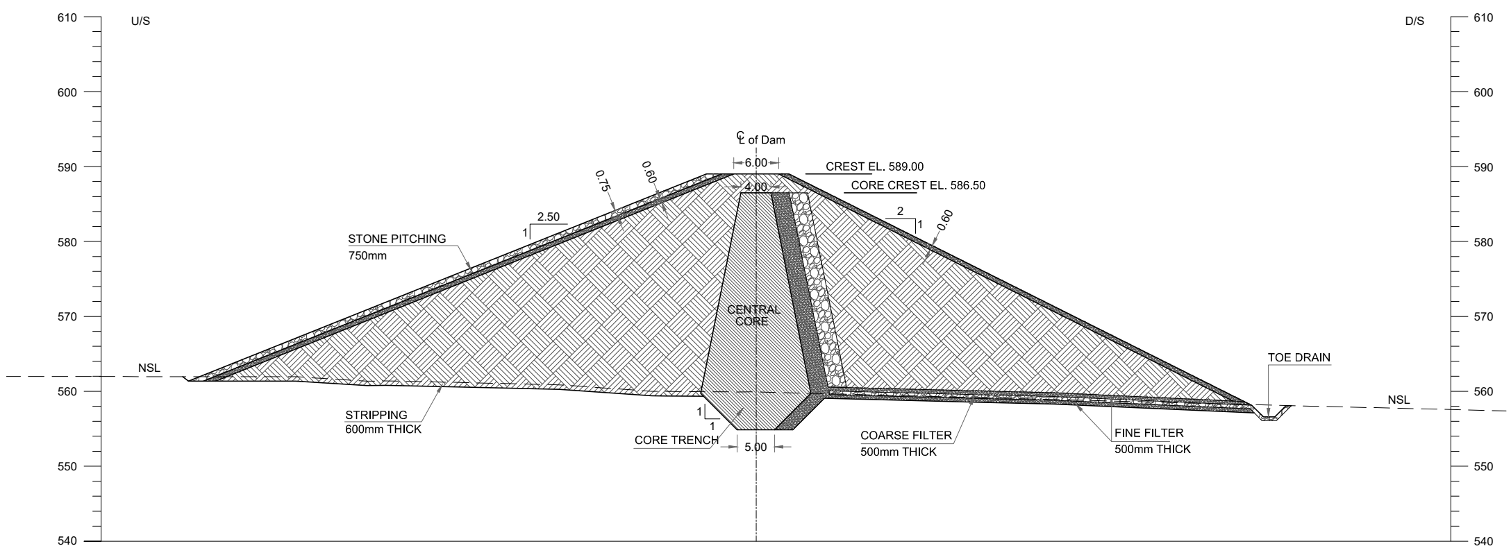
RD 0+100
