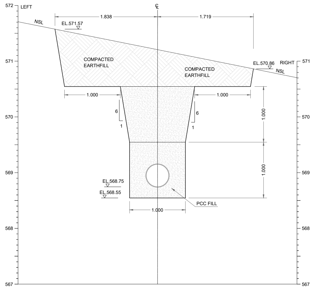
RD 0+020
