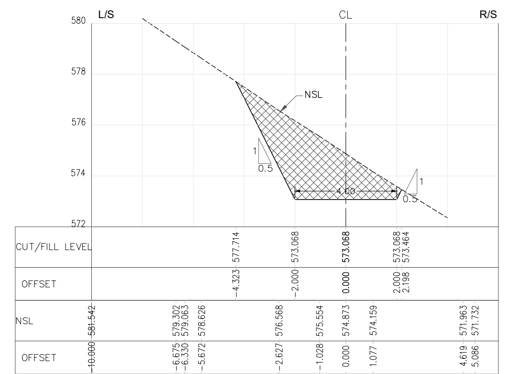
RD=0+650.000
