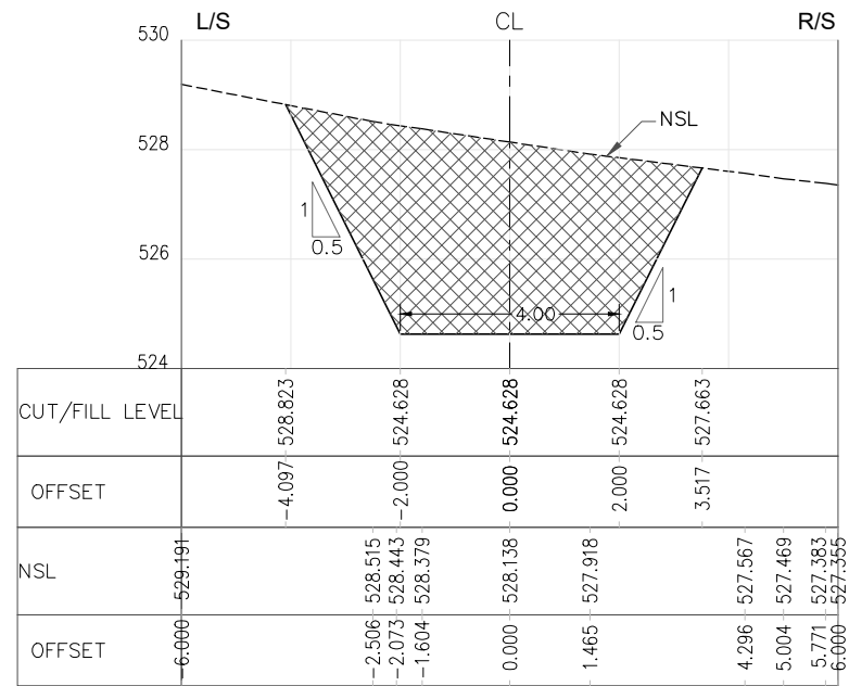
RD=2+700.000
