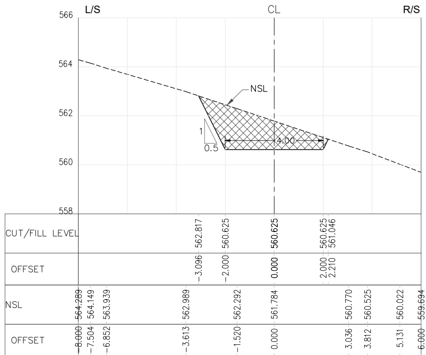
RD=1+600.000
