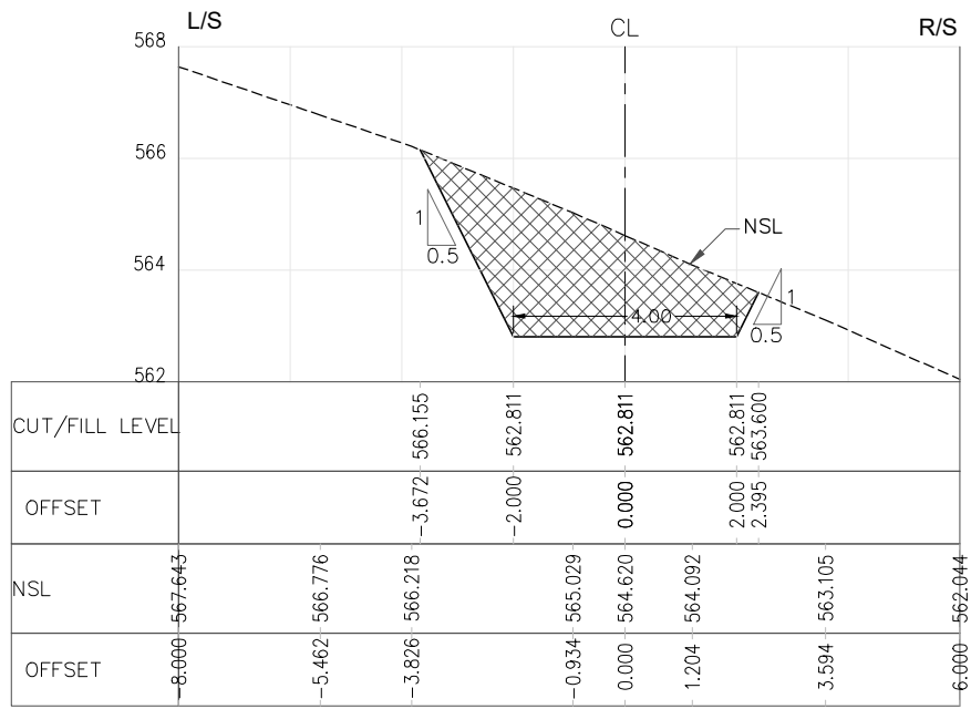
RD=1+500.000
