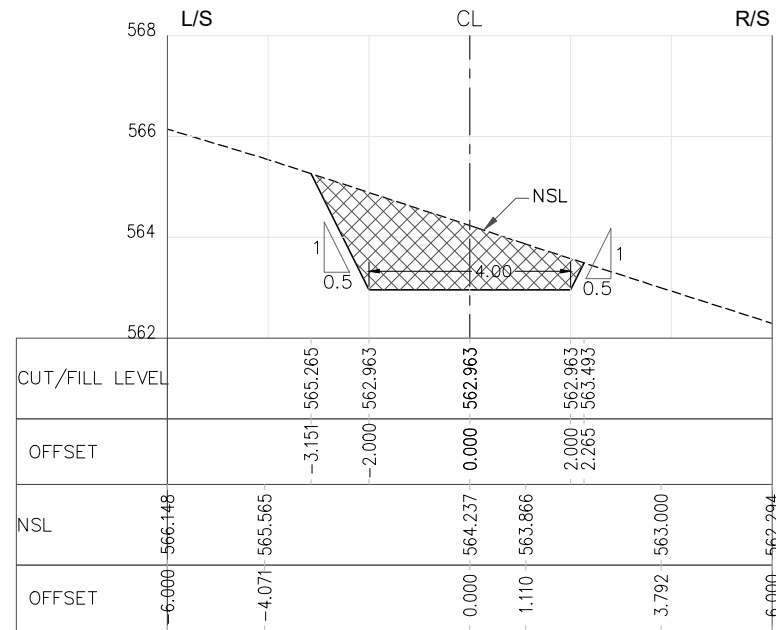
RD=1+250.000
