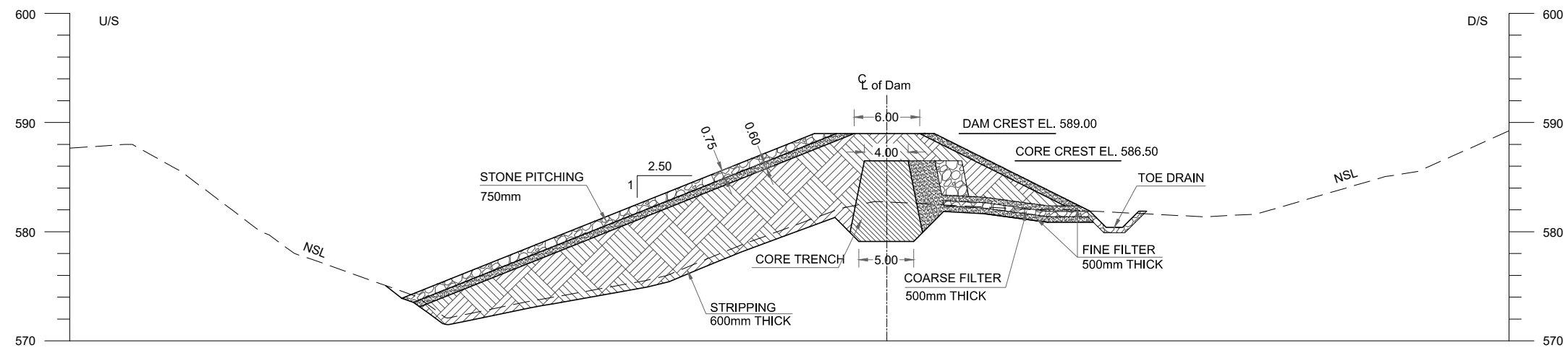
RD 0+270
