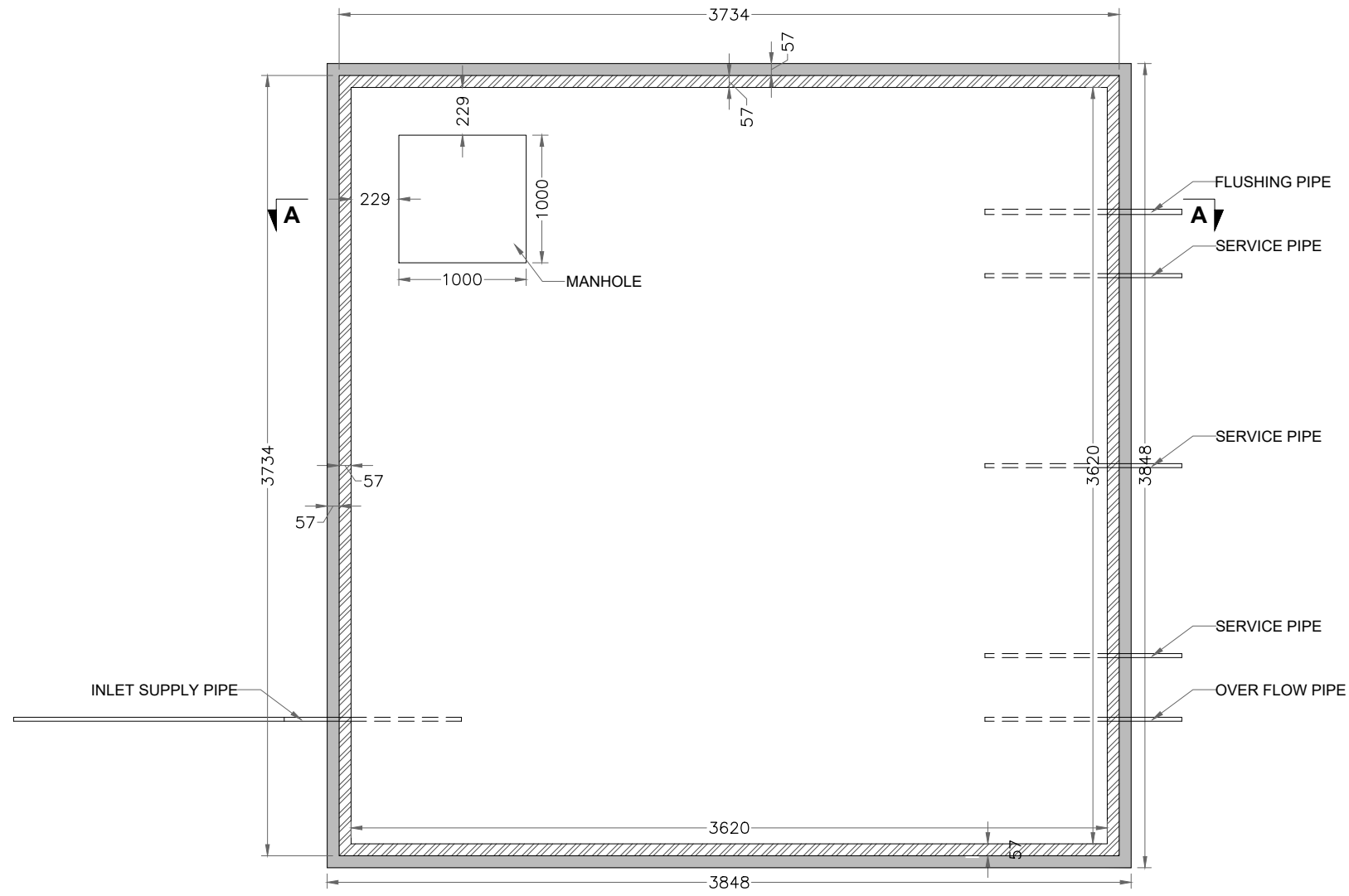
PLAN SCALE: 1:30
