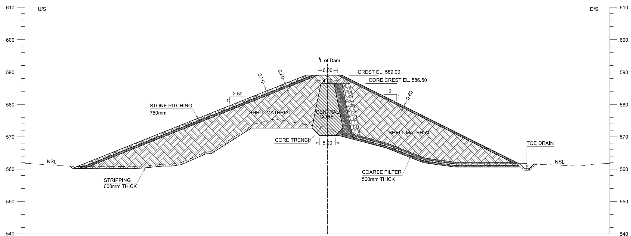
RD 0+180
