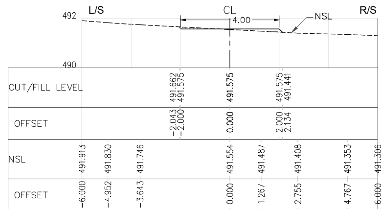
RD=3+800.000
