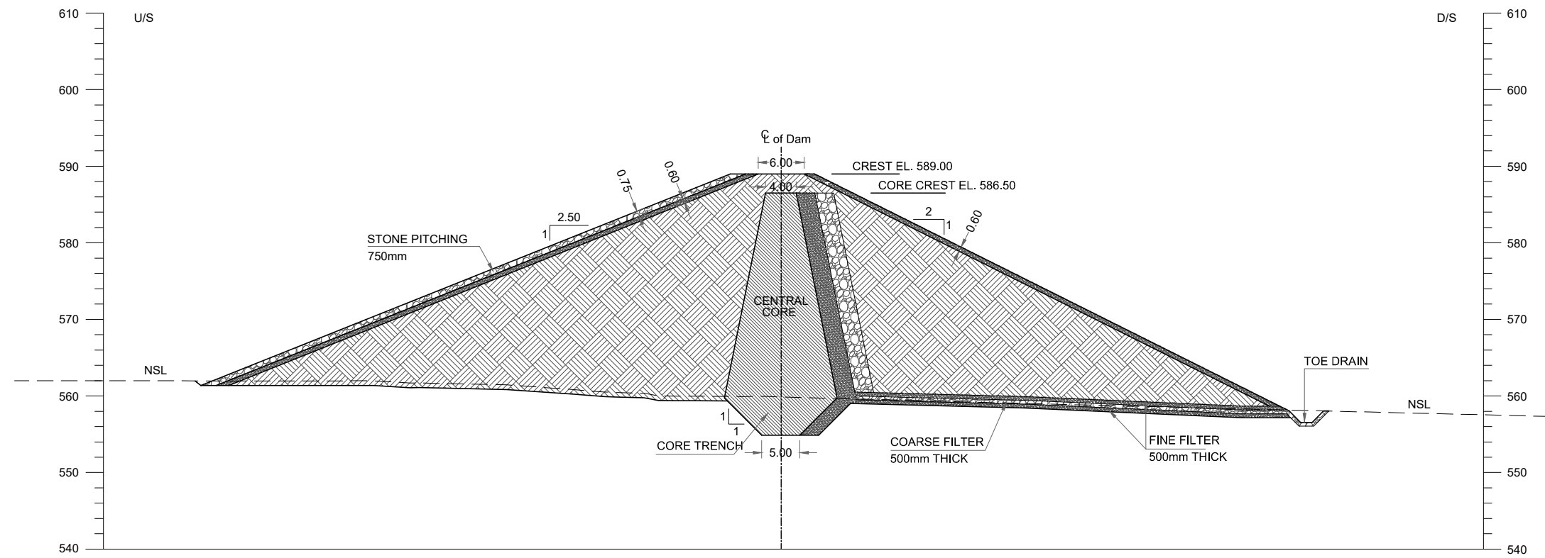
RD 0+090
