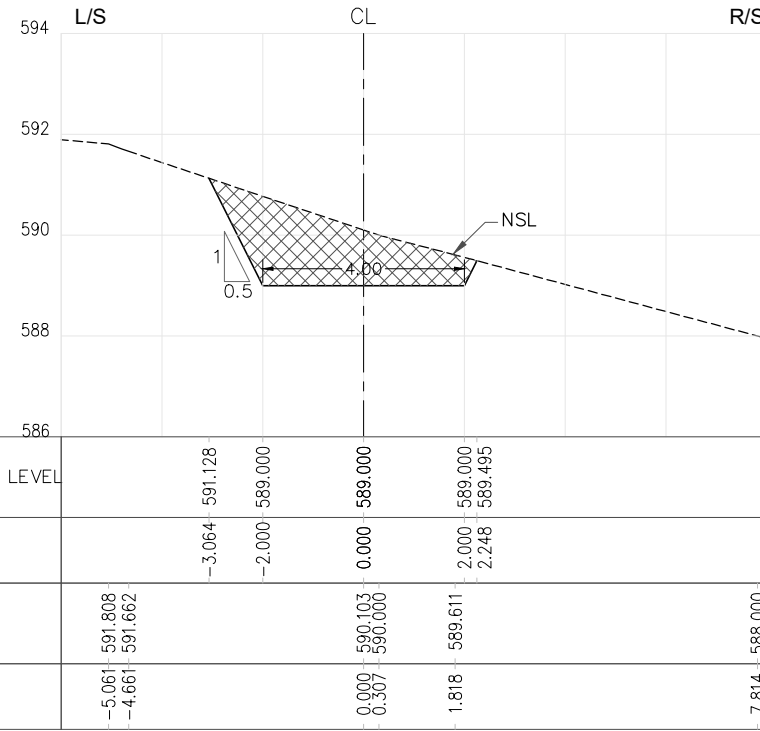
RD=0+050.000
