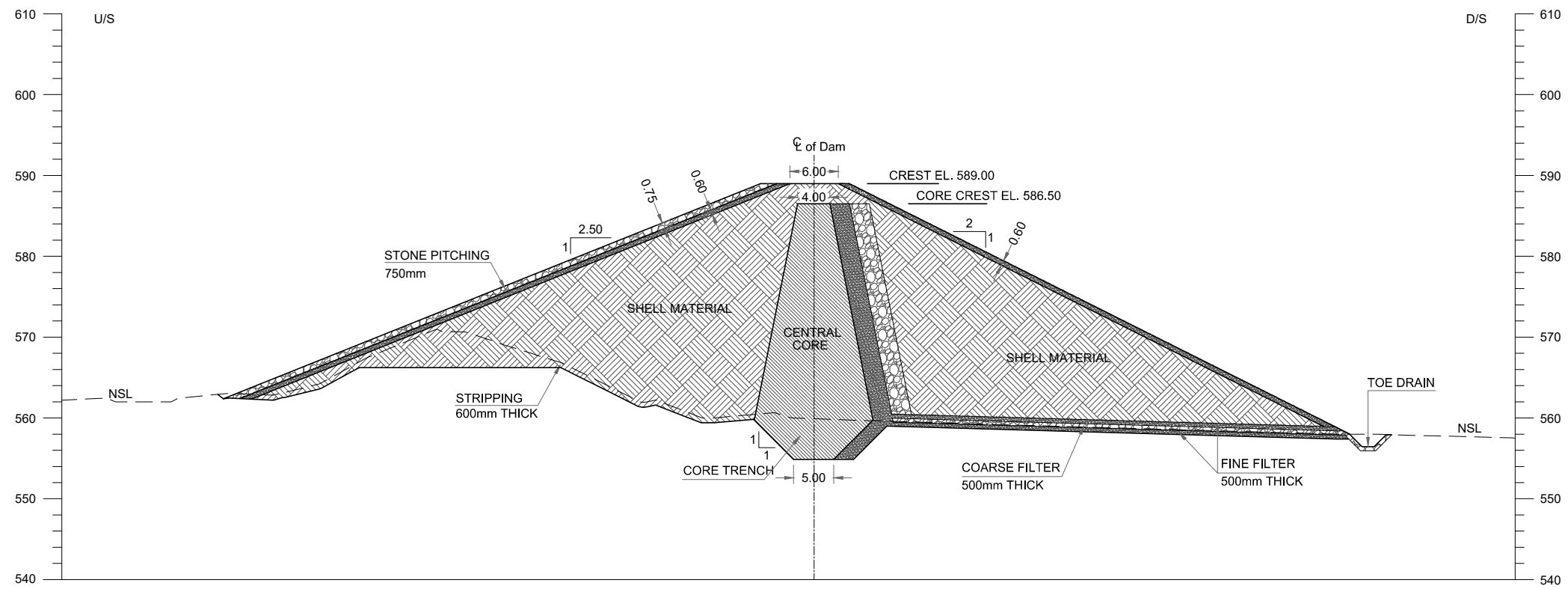
RD 0+070
