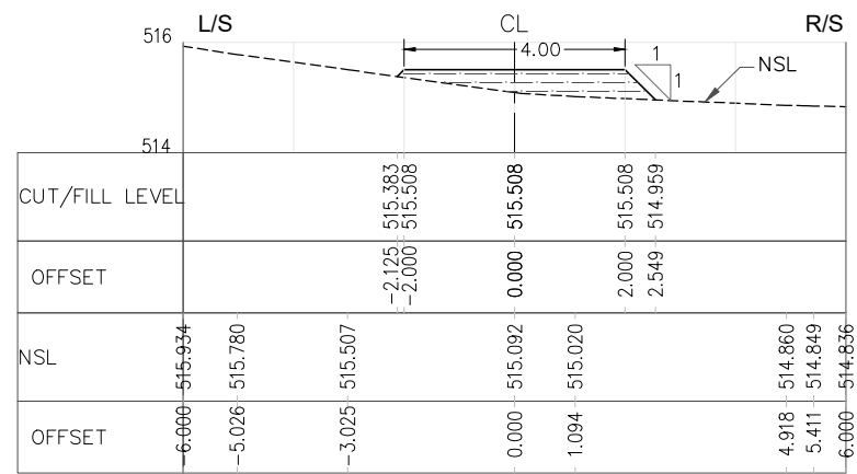
RD=3+000.000
