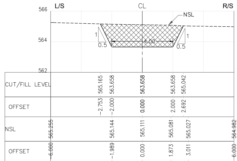
RD=1+200.000
