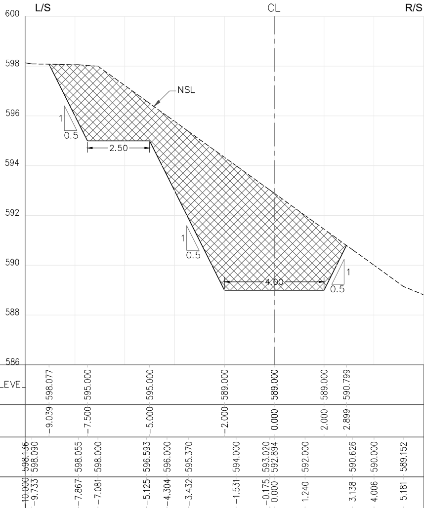
RD=0+100.000
