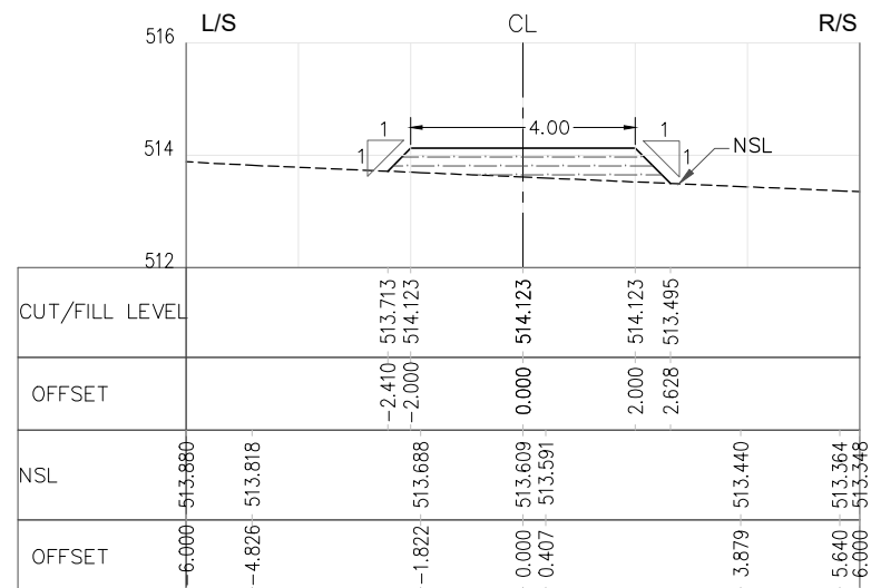
RD=3+100.000
