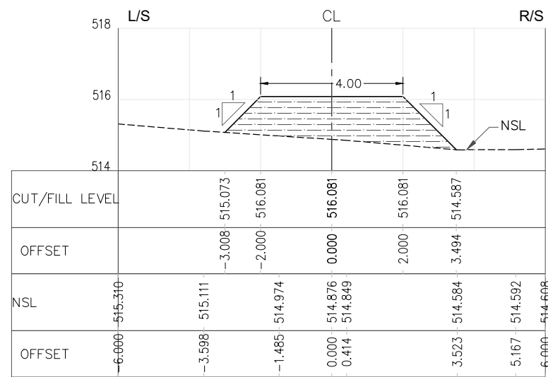
RD=2+850.000
