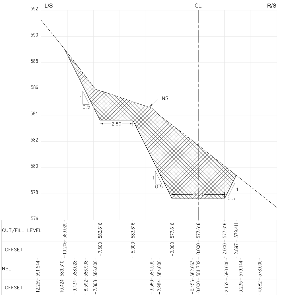
RD=0+550.000
