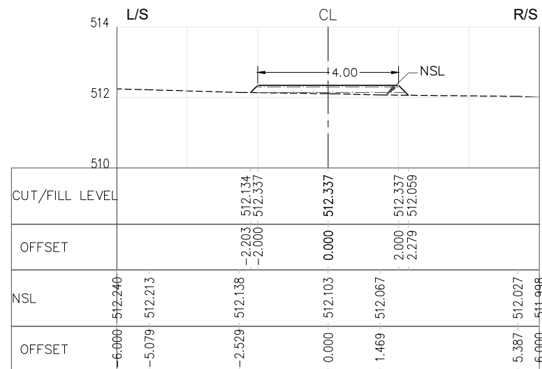
RD=3+150.000
