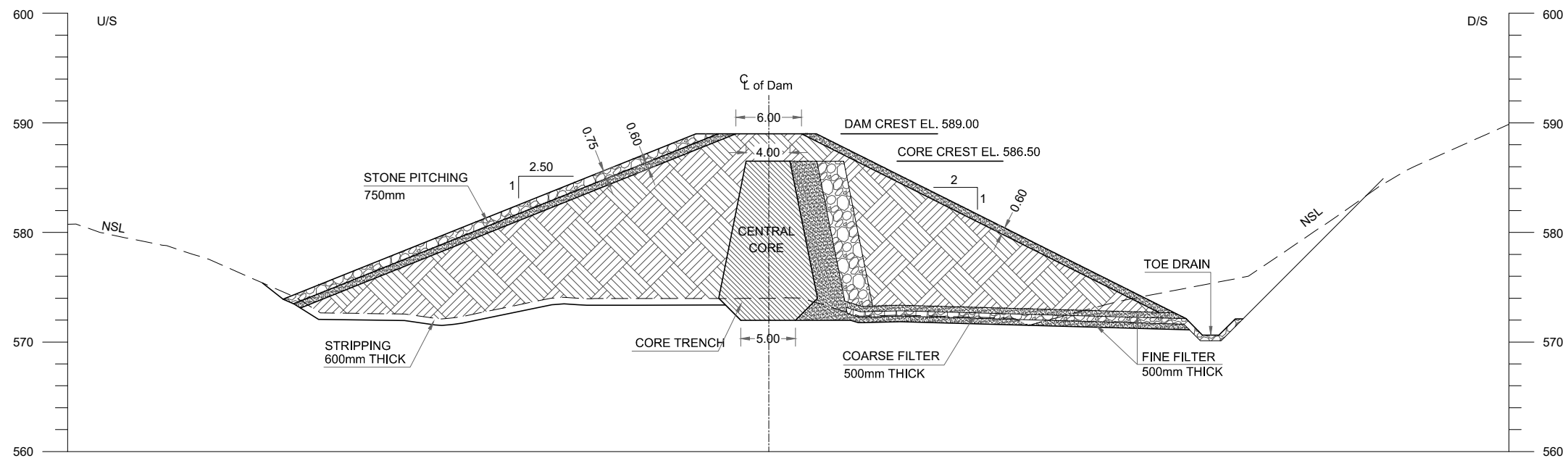
RD 0+250
