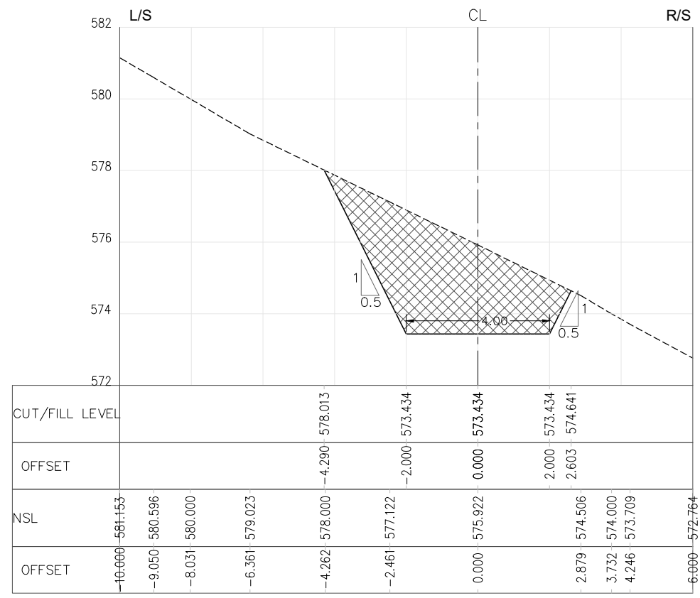
RD=0+100.000
