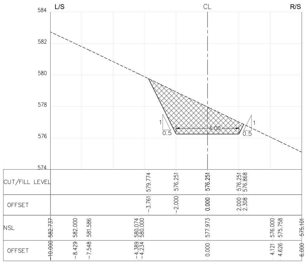
RD=0+150.000
