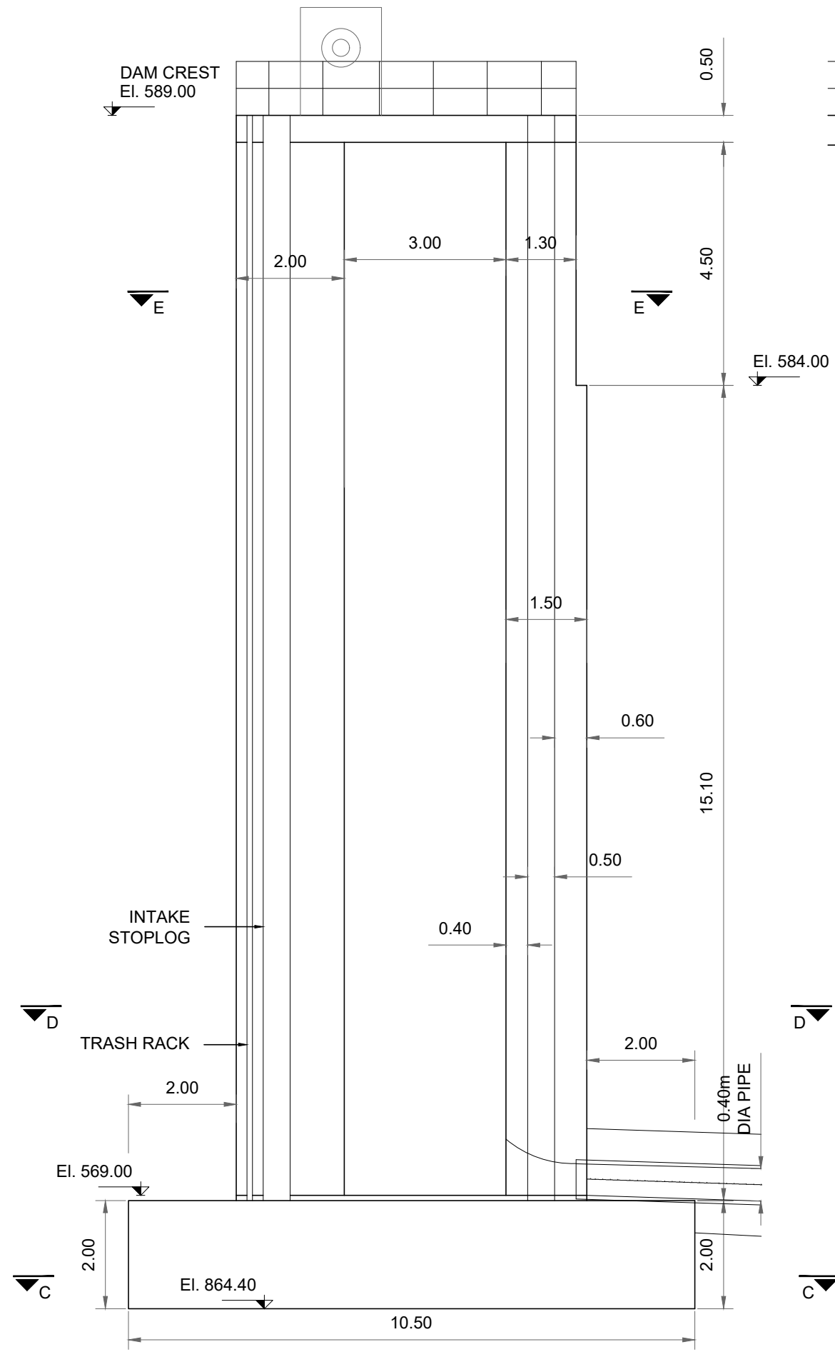
SECTION A-A
