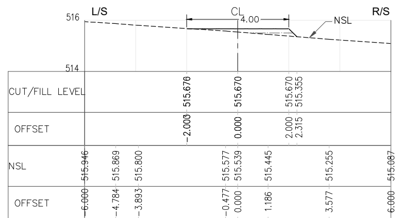
RD=2+900.000
