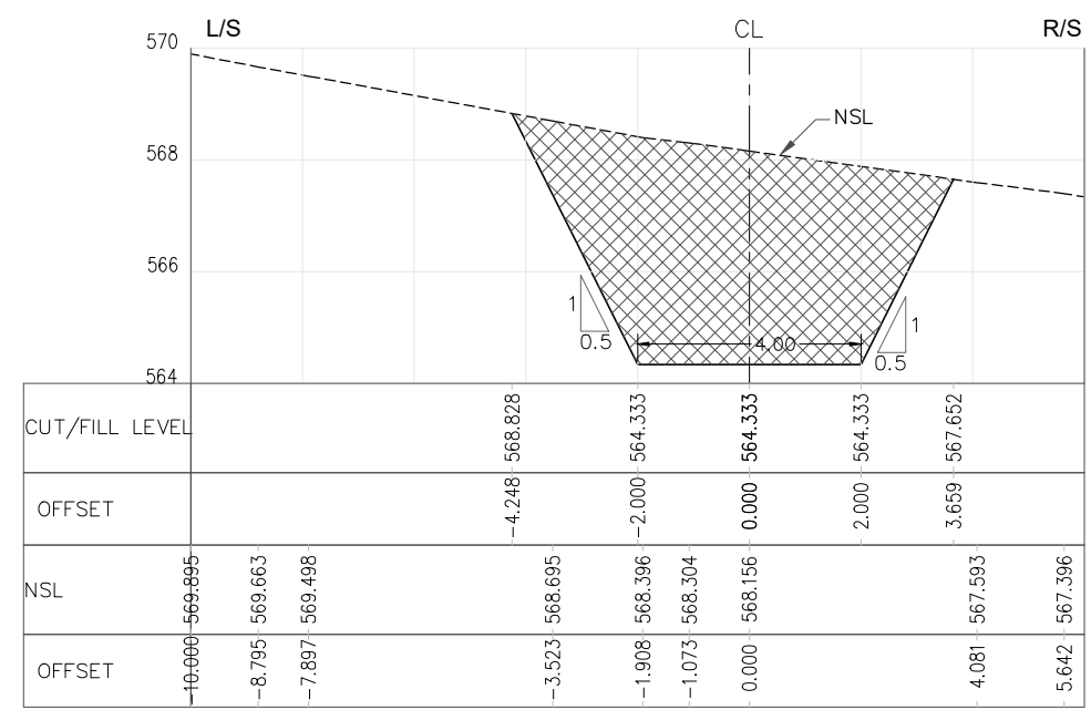
RD=0+850.000
