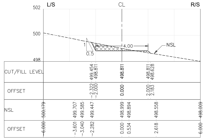
RD=3+600.000
