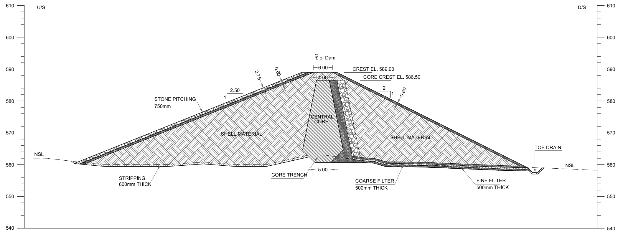
RD 0+150
