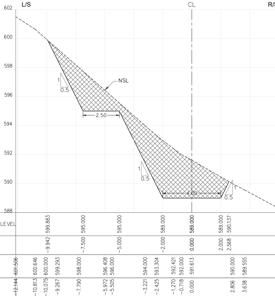
RD=0+150.000
