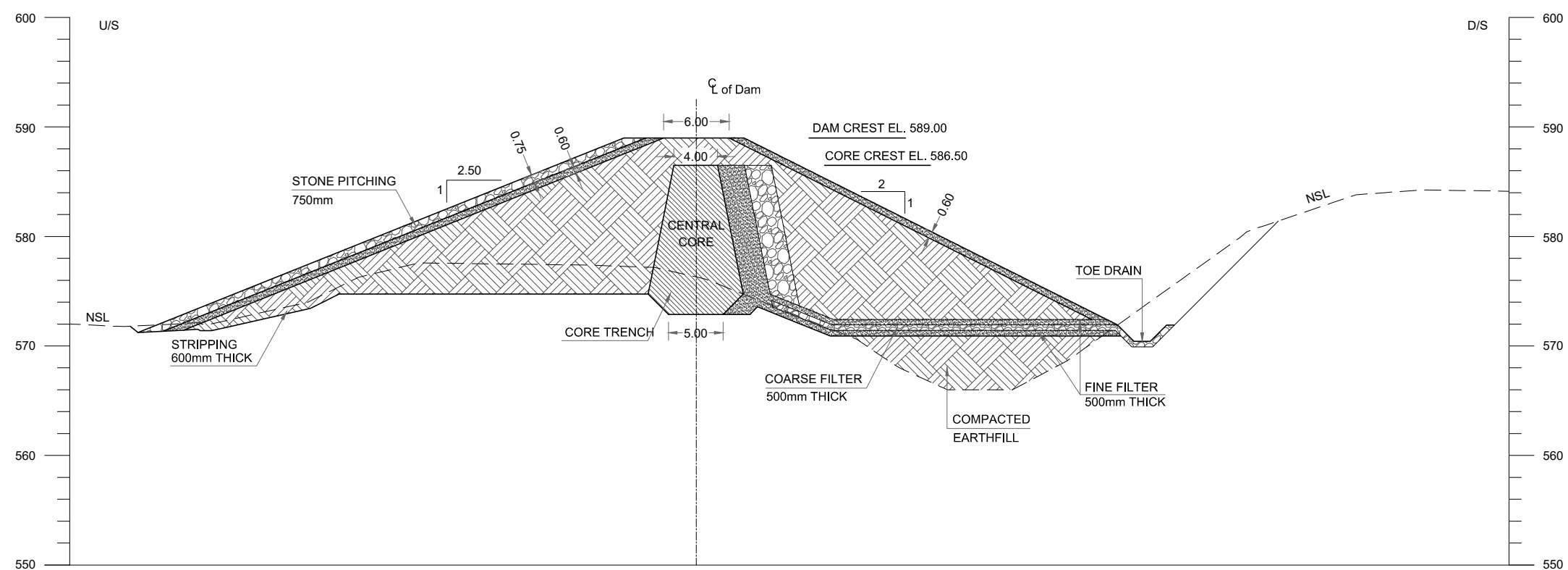
RD 0+230
