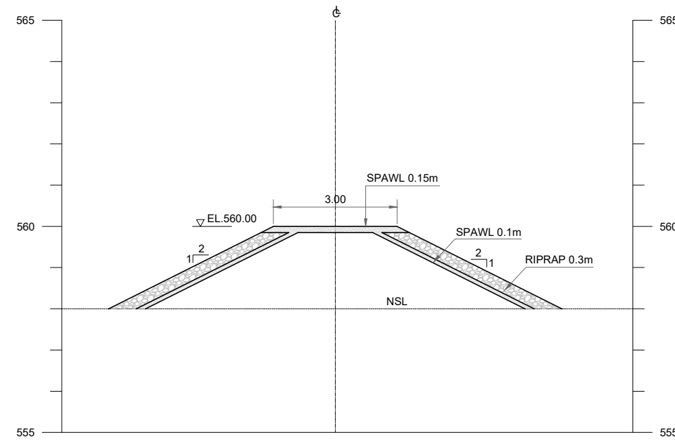
B-B
