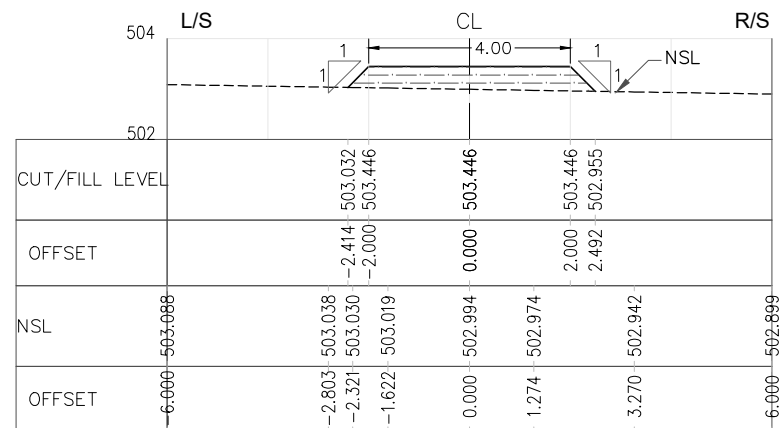
RD=3+500.000
