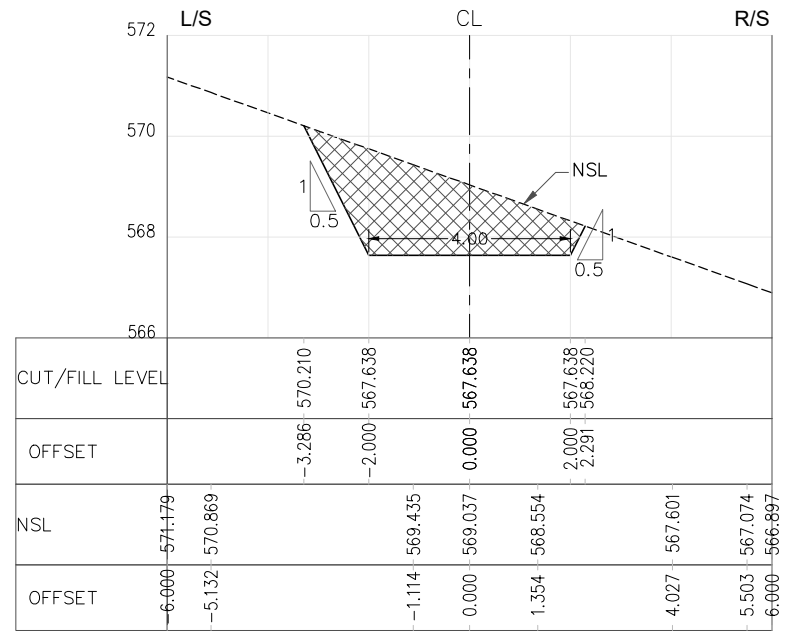
RD=0+950.000
