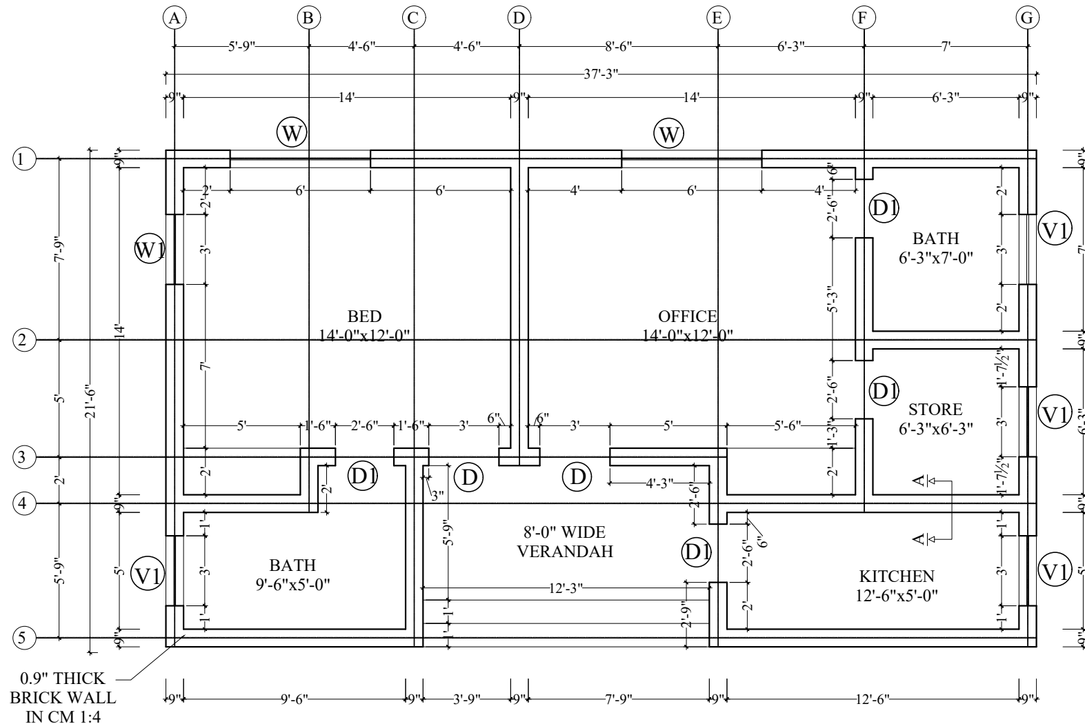
PLAN 750 sft
